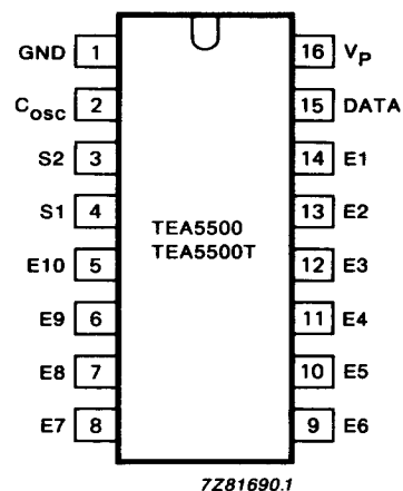
Fig. 2 Pinning diagram.
